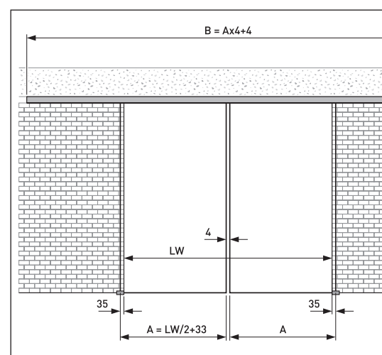
Montage au plafond 2 vantaux , en ensembles individuels d'une largeur de vantail allant jusqu'à 975 mm ou 1475 mm, longueurs de stock.
