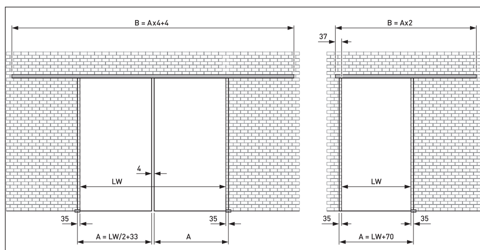
Montage mural 2 vantaux , en ensembles individuels d'une largeur de vantail allant jusqu'à 975 mm ou 1475 mm, longueurs de stock.
